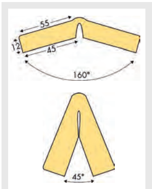
Kantenschutz Flex, Winkel, Typ H+
