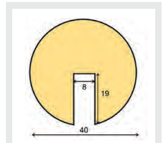
Profilschutz Kreis, Typ B
