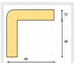
Kantenschutz Winkel, Typ H+
