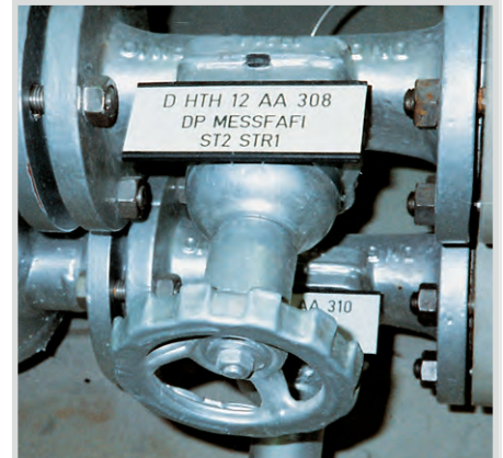
Schilderträger aus ABS ohne Endkappen
