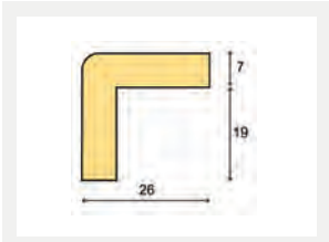
Kantenschutz Winkel, Typ E
