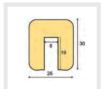
Profilschutz Viereck, Typ G
